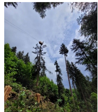
Abbildung 7 Laufkatze über dem Arbeitsplatz
